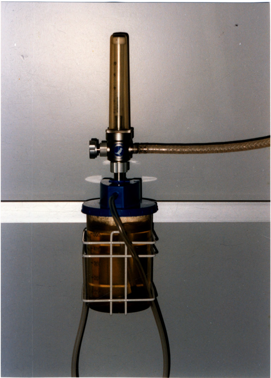
Устройство для увлажнения кислорода при ингаляции УК
